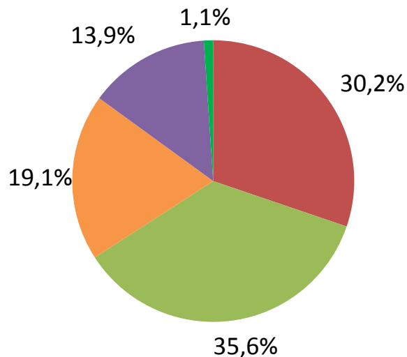
Emissions GEH 2014
