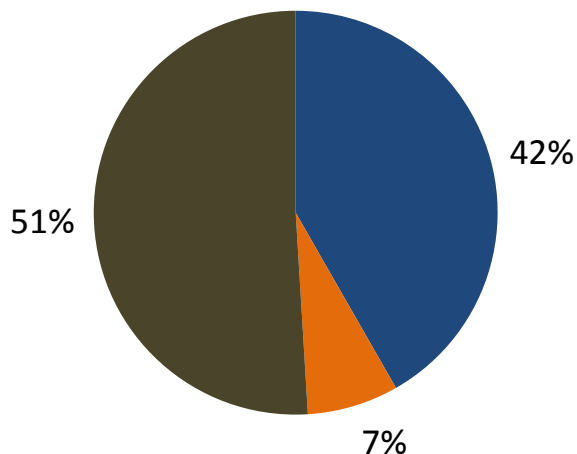
Emissions GEH 2010
