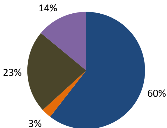
Emissions GEH 2010
