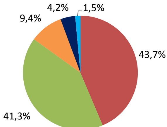
Emissions GEH 2014
