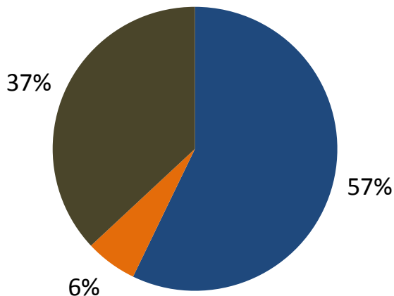
Emissions GEH 2010
