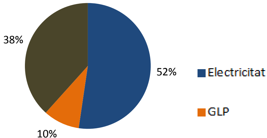
Emissions GEH 2014
