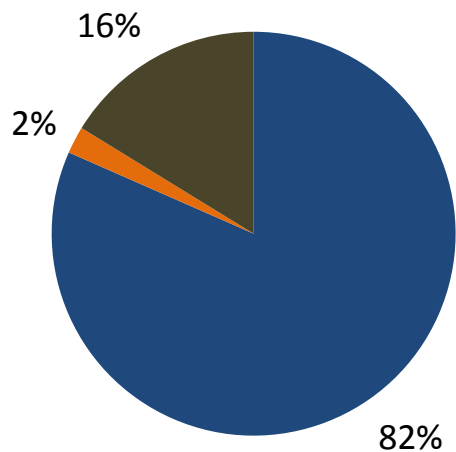
Emissions GEH 2010
