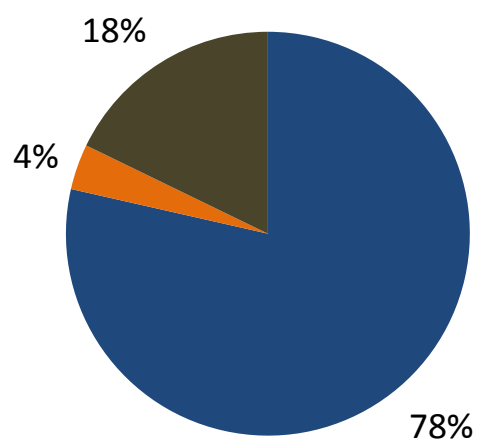
Emissions GEH 2014
