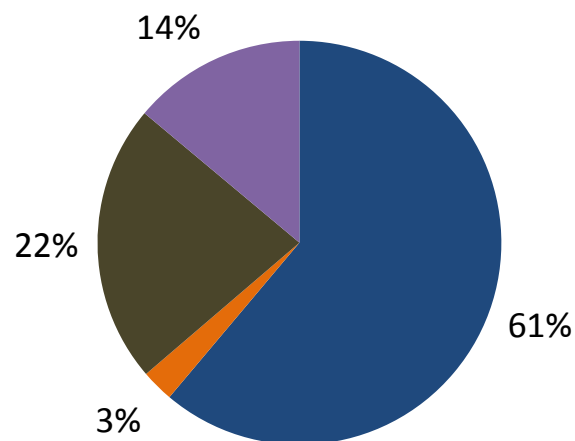
Emissions GEH 2014
